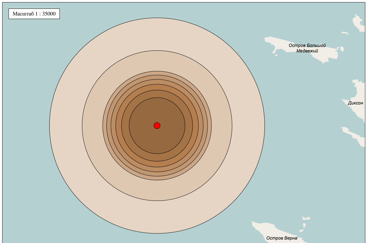
Рис. П8.1. Схема распространение нефтяного пятна при разливе 1113,55 \text{ м}^3 легкого топлива у о. Диксон на входе в Енисейский залив (С15.9)
